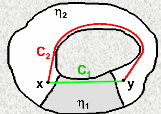
C_2 est le plus court chemin
