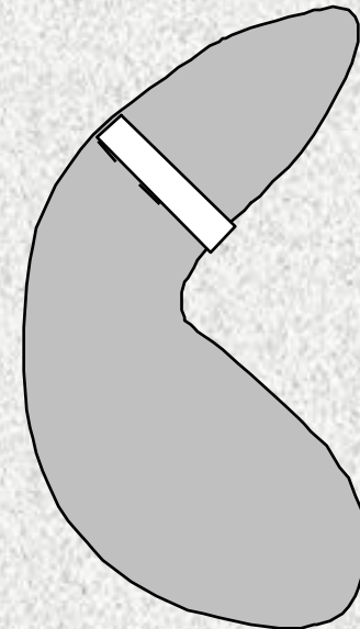
X \cup \varepsilon(X^c \cup Y)
