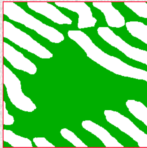
Particules touchant les bords
